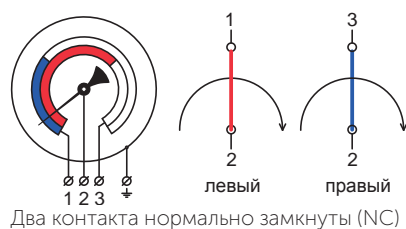
Исполнение III ЛРПР (левый размыкающий контакт, правый размыкающий)
