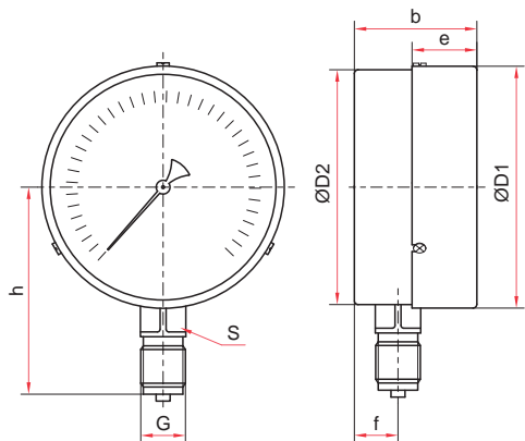
Радиальное присоединение
