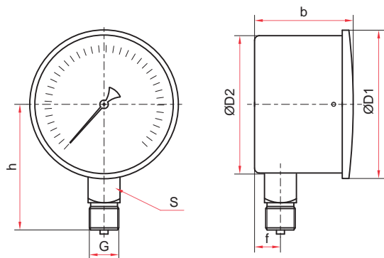
Радиальное присоединение
