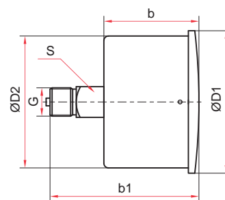
Осевое присоединение
