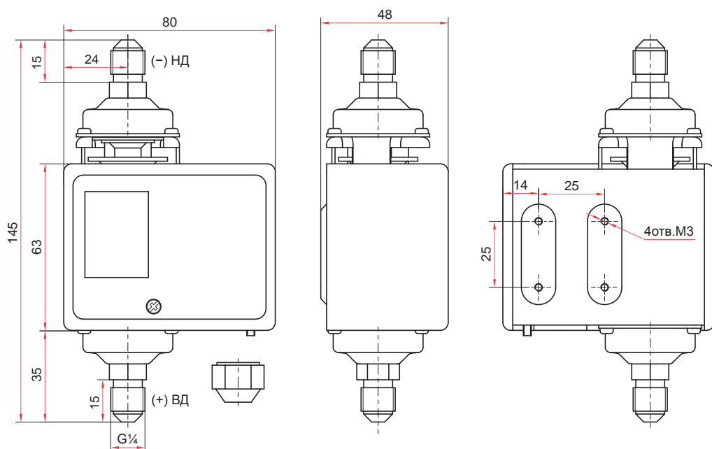
Дифференциальное реле давления РДД-2Р
